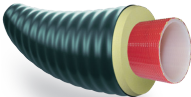
ТВЭЛ-ПЭКС-К (с армирующей системой)
